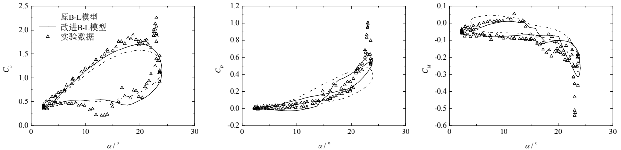
图 6 S809 翼型的动态气动力仿真结果与实验数据的对比, \alpha = 14 + 10\sin(\omega t) , k = 0.1 , M = 0.08
