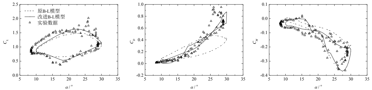
图 7 S809 翼型的动态气动力仿真结果与实验数据的对比, \alpha = 20 + 10\sin(\omega t) , k = 0.078 , M = 0.1
